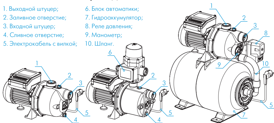
Поверхностный насос
