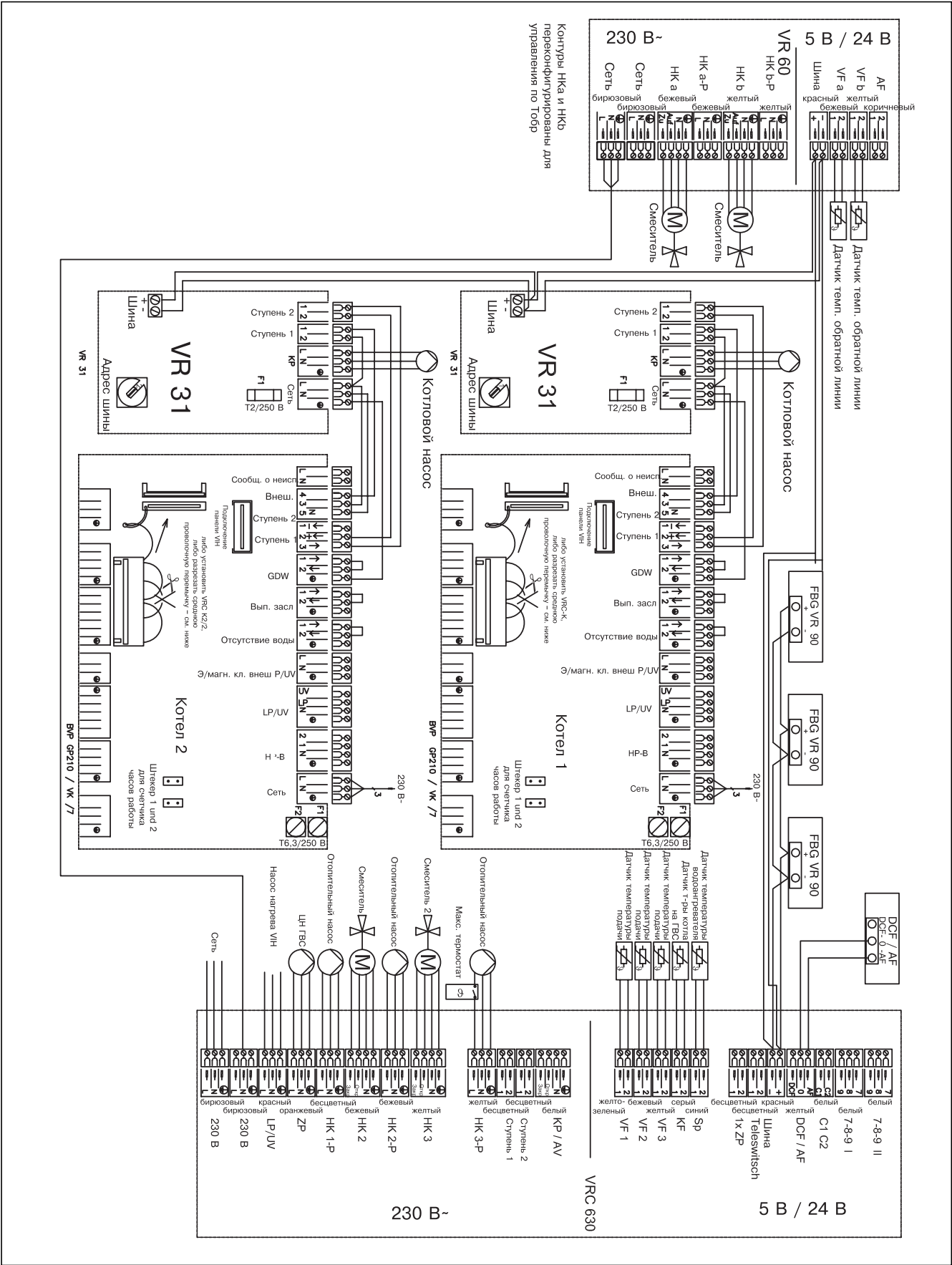
Рис. 4.15 Соединительная электропроводка VRC 630, GP210, 3 OK, V1H
