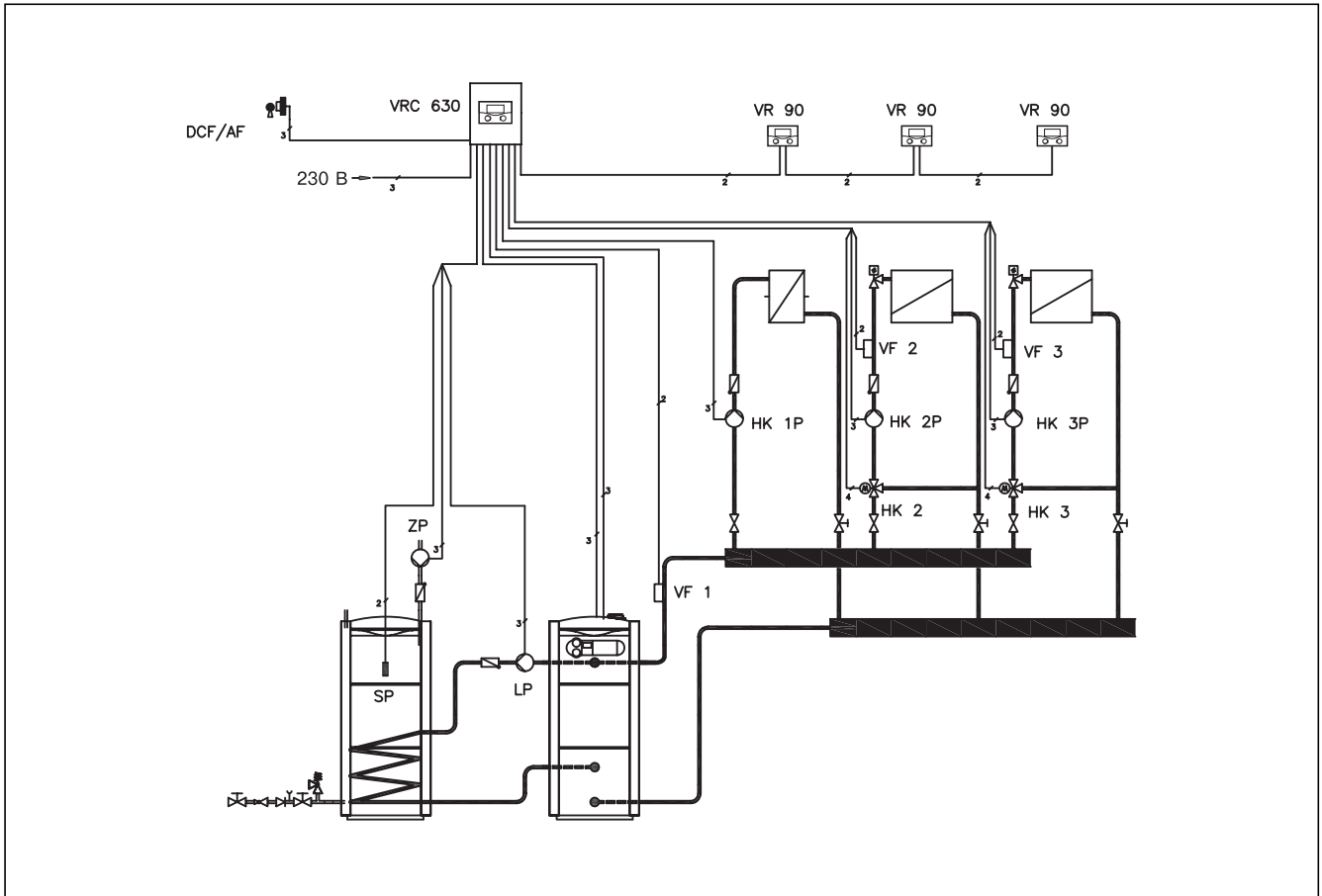
Рис. 4.10 calorMATIC 630 напольный прибор 1
