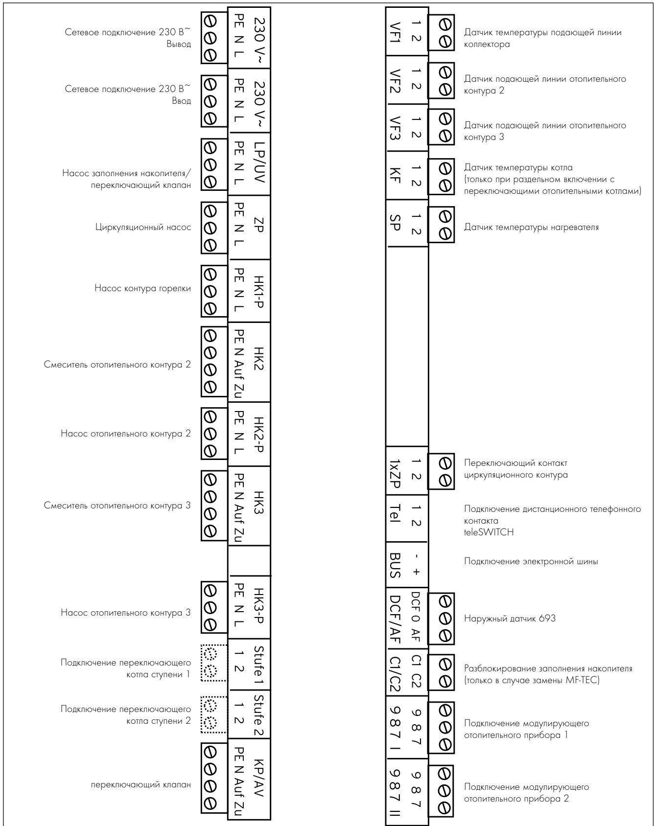
Рис. 4.3 Разводка контактов
