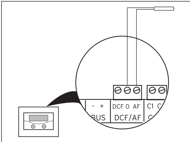
Рис. 4.16 Подключение VRC 693
