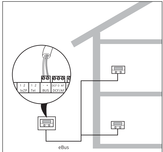
Рис. 4.17 Подключение приборов дистанционного управления
