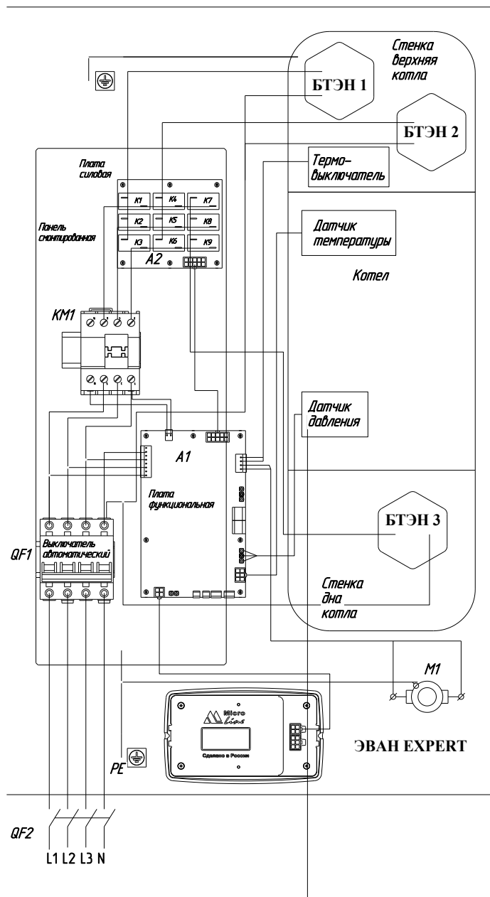
Рис. 12 Схема подключения ЭВАН EXPERT.
